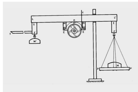
Schéma du dispositif d'essais de G.A.Hirn (1854)
